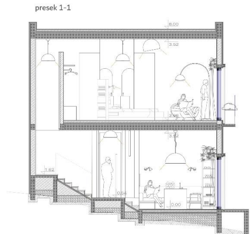
Slika 9. Karakterističan presek
